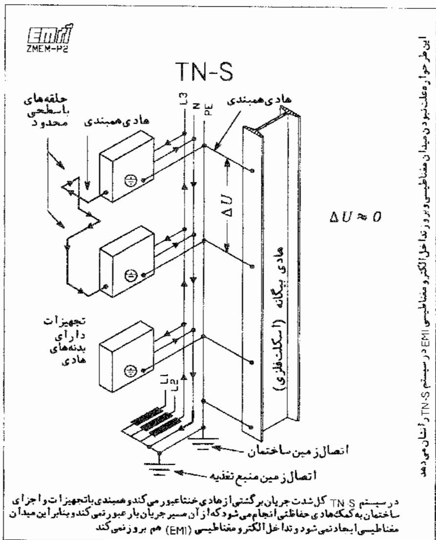
شکل 4P2-2 نحوه حرکت جریانهای برگشتی از هادی N بدون استفاده از مسیرهای اضافی
