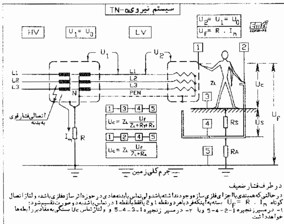
شکل 4-AP2 برقرگرفتگی در حالتی خصوصی با اتصال زمین مشترک حفاظتی - ختا در سیستم TN
