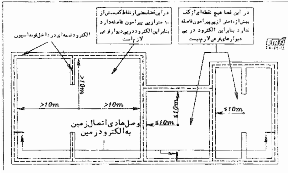
شکل ۲۲- 4PI- الکترو دهای نصب شده در فونداسیون
