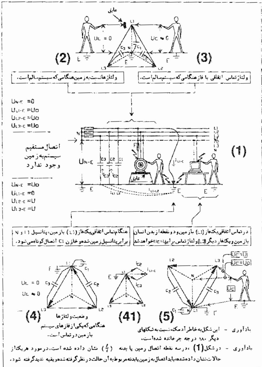
شکل ۱-۳۳۱ یک سیستم توزیع الکتریکی ابتدایی که اتصال به زمین ندارد (این سیستم پیش درآمد سیستمی است که امروزه II خوانده می شود)
