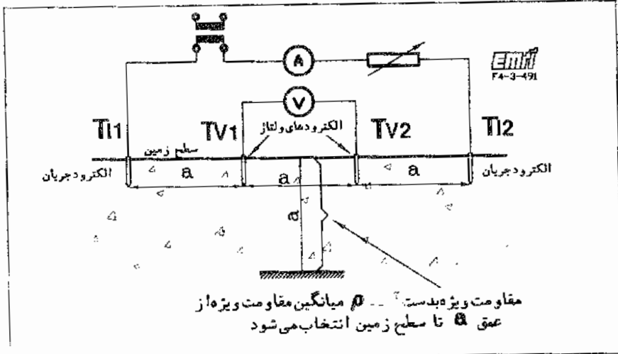
شکل ۱-۴۹۲ نحوه استقرار الکترودها و وسایل اندازه‌گیری برای مقاومت ویژه
