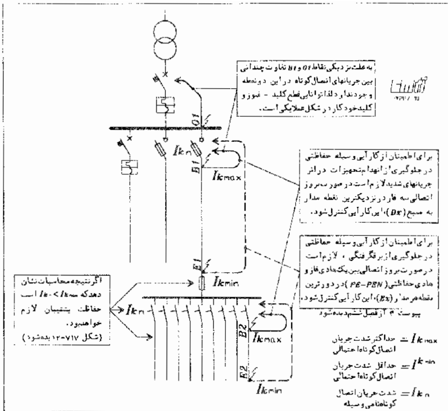
شکل ۷۱۷-۱۰ بعضی از مسائلی که باید در محاسبه حداکثر و حداقل جریانهای اتصال کوتاه منظور شوند.
