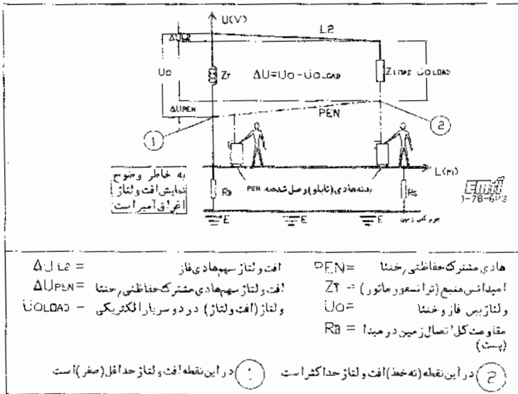
شکل 6P3-2. افت ولتاژ در هادی فاز L2 و هادی مشترک حفاظتی رعایت PEN در حالتی که سطح مقطع هادی
