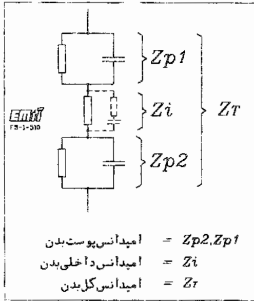
شکل ۱-۵۱۰ اجزای سازنده مقاومت بدن
