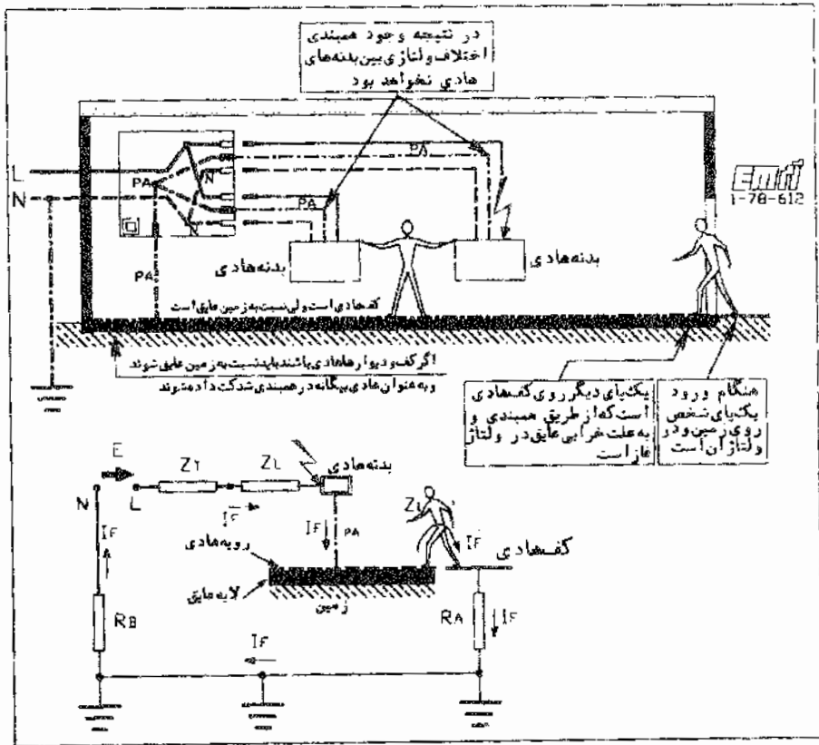
شکل ۶-۶۲۲ حفاظت در برابر تماس غیر مستقیم با استفاده از همولتاژ کتنه بدون اتصال به زمین
