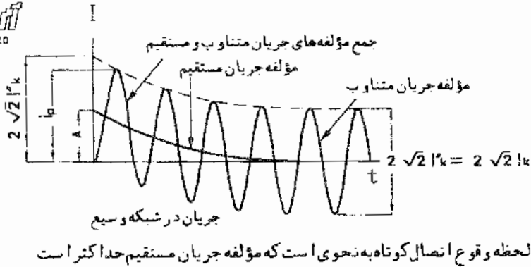
شکل ۷-۱۷-۲ اوسیلوگرام یک اتصال کوتاه با حداکثر جابجایی (حداکثر مؤلفه جریان مستقیم)
