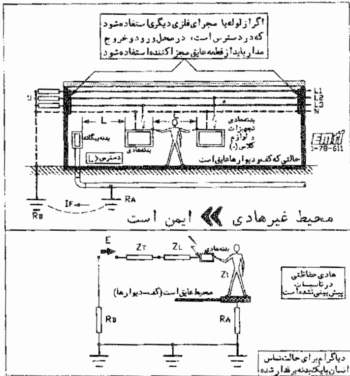
شکل ۲۲-۵ شرایط تأمین ایمنی به کمک محیط عایق با استفاده از تجهیزات کلاس (۰)
