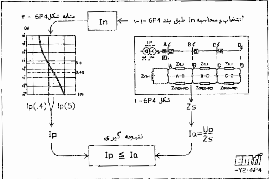
شکل 6P4-5 خلاصه نحوه کنترل کارایی سیستم با استفاده از منحنیهای فیوزها (روش صحیح انجام کار)
