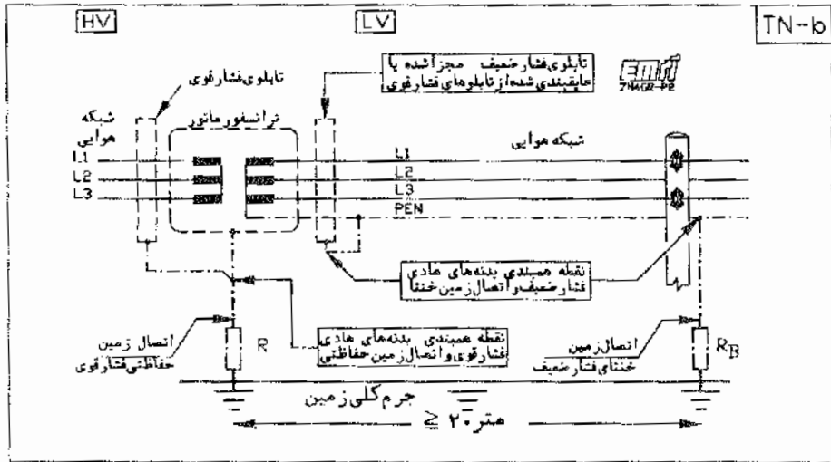
شکل 4P2-10 حالتی با دو اتصال زمین مجزا - خط هوایی و زمین تابلو از طریق PEN در سیستم TN
