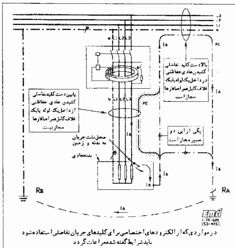
شکل ۶۲۱-۱۳ نحوه استفاده از یک کلید حفاظتی جریان تقاضایی در صورت وصل به الکترود اختصاصی
