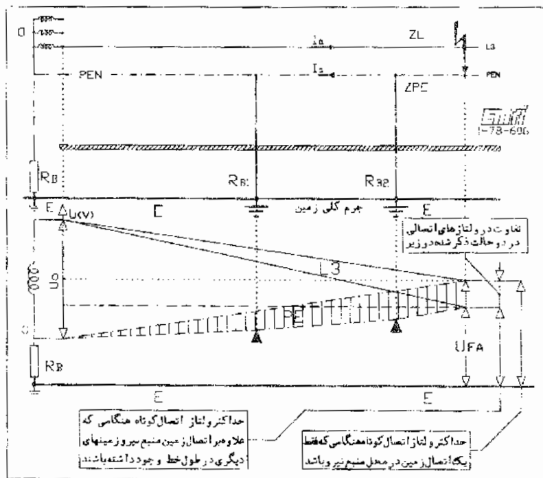
شکل ۶۲۱-۷ نحوه اثر اتصال زمین مکرر در ولتاژ اتصال و در نتیجه ولتاژ برگرفتنی
