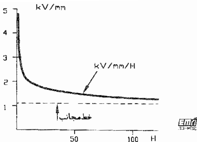
شکل ۱۰-۳۱۱ استانداردگی عایق در برابر تنش میدان الکتریکی نسبت به زمان (منحنی نوعی)
