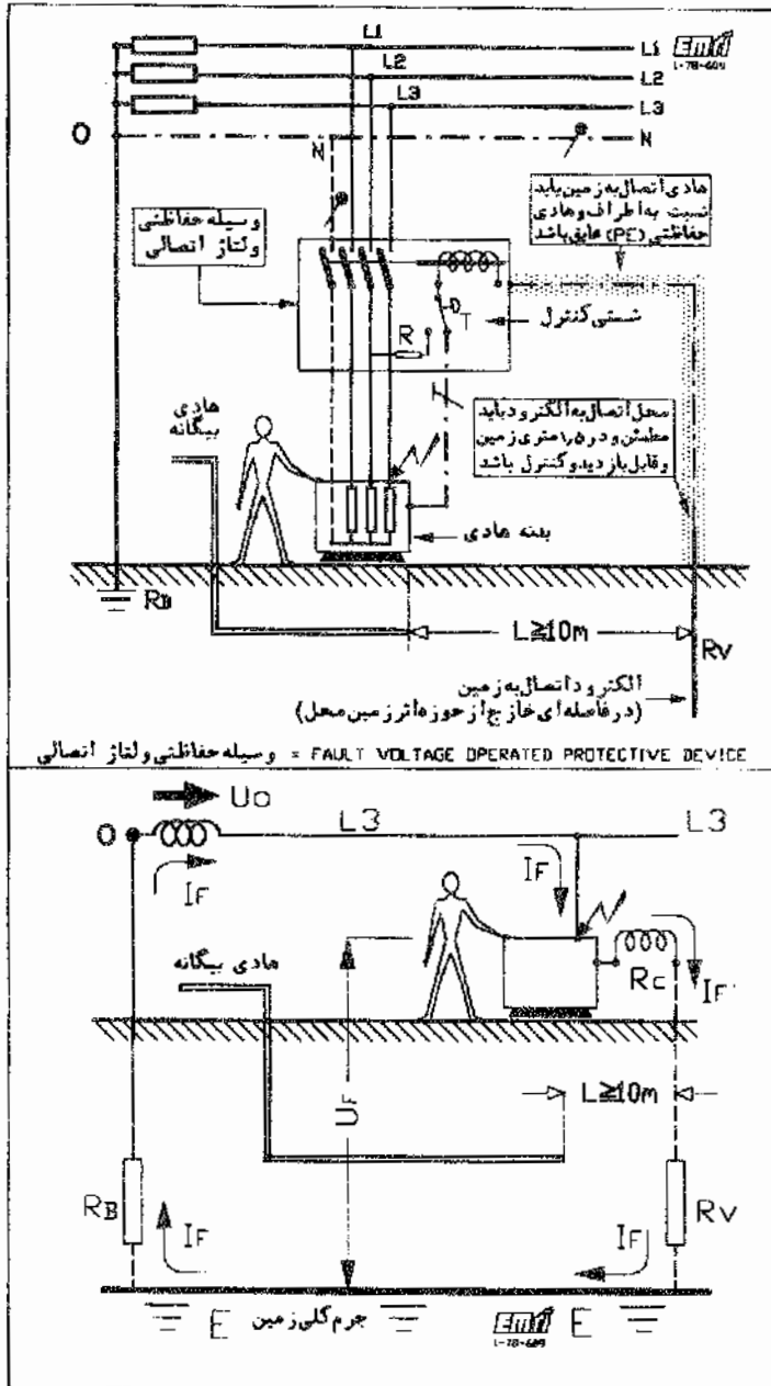
شکل 6-1 نحوه استفاده از وسایل حفاظتی و لنای اتصالی
