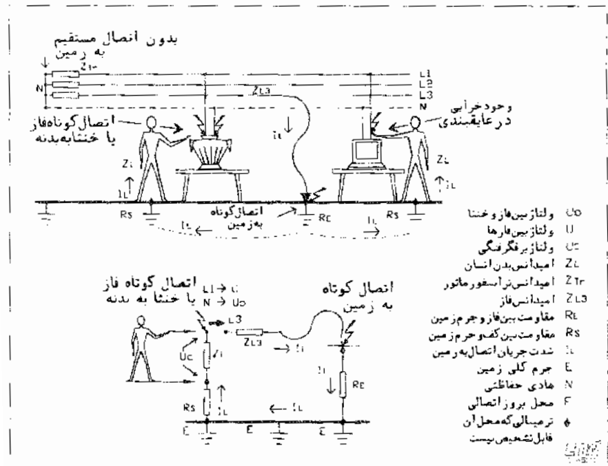
شکل ۲-۳۲۱ سیستم توزیع ابتدایی (بدون اتصال به زمین سیستم) که در آن تجربه مدار اتصال کوتاه در دو حالت مختلف نشان داده شده است.
