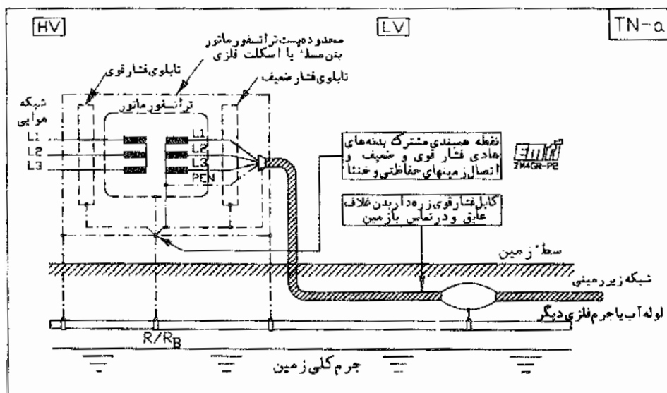
شکل 9-4P2 حالتی برای احداث اتصال زمین مشترک اگر احداث زمینهای مجزا ممکن نباشد. در سیستم TN
