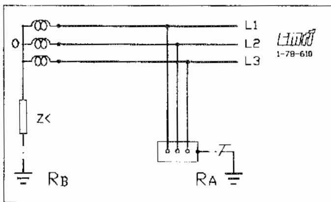
شکل ۱۴-۶۲۱ (۲) سیستم IT نوع وصل به زمین از طریق امپدانس ساده
