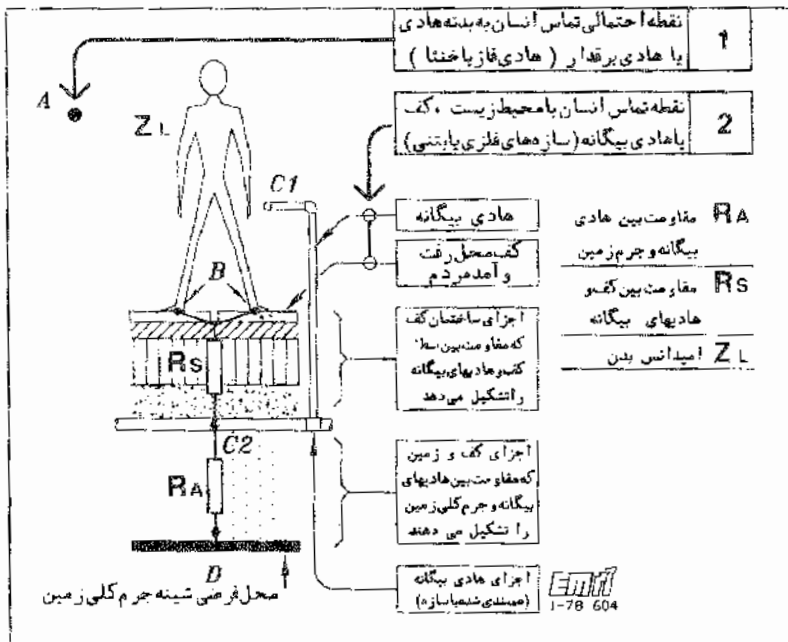
شکل 6PI-۱ وضعیت فیزیکی در قبل از بروز برق‌گرفتگی - ساختار مقاومتها
