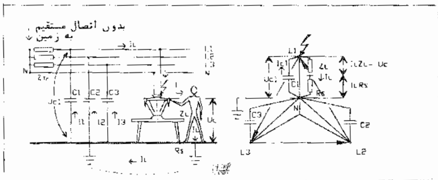
شکل ۲-۳۲۱ سیستم توزیع ابتدایی (بدون اتصال به زمین سیستم) که در آن متفاوتهای اتصال زمین دیگر منظور شده اند.
