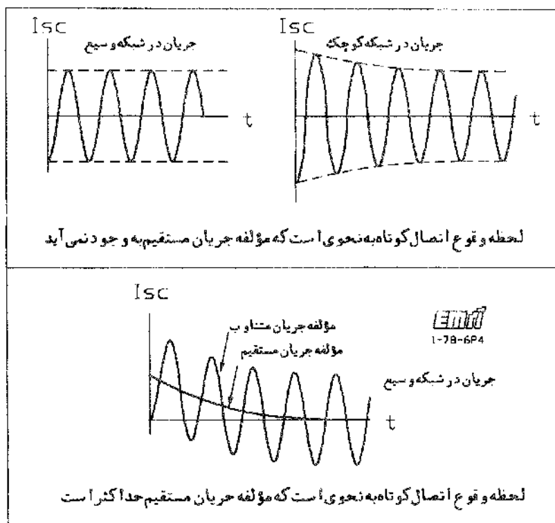
شکل 6P4-7 لوسیلوگرامهای حالتیهای مختلف جریان بسته به لحظه وقوع اتصال کوتاه و نوع شبکه
