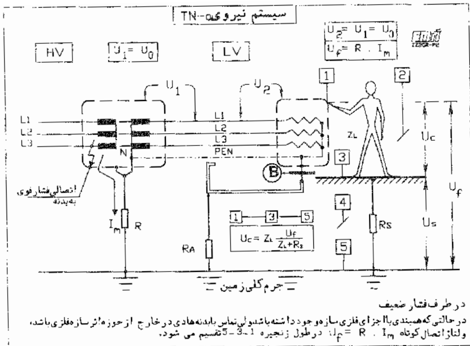
شکل 4P2-5 برقرنگی در یک حالت خصوصی با اتصال زمین مشترک حفاظتی - ختا در سیستم TN
