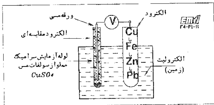
شکل 4PI 11 پتانسیل نسی فلزات در الکترو لیت (زمین)
