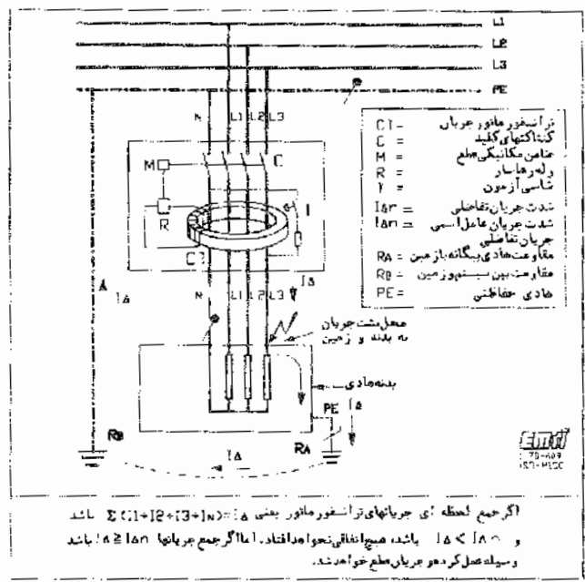
شکل ۳-۳۳۲ طرحواره یک وسیله (کلید) حفاظتی جریان نفاذی
