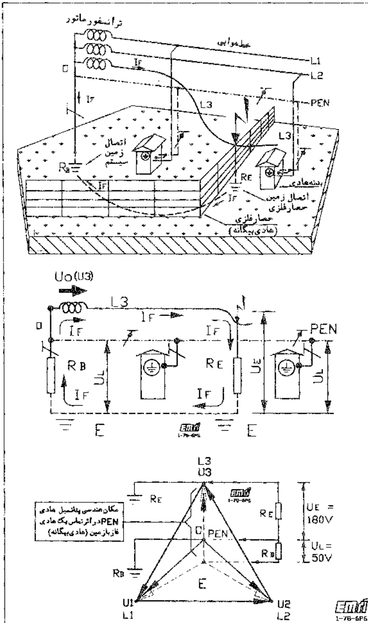
شکل 1-6P6 و ضمیمه که در اثر اتصال کوتاه بین یک فاز و یک هادی بیگانه که در همبندی شرکت ندارد (خارج از
