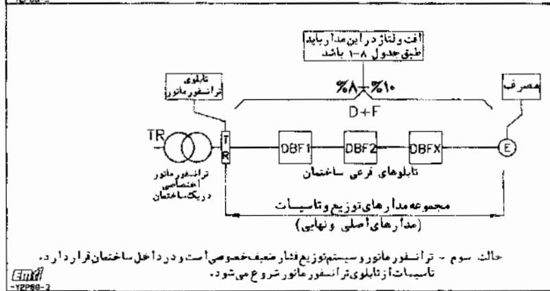
شکل ۲-۸-۱ طرحواره حالتهای مختلف تقسیم افت ولتاژ در مدارهای مختلف
