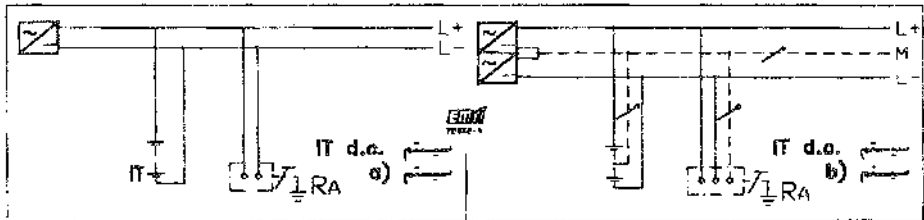
شکل ۲۱۸-۵ سیستم IT d.c.
