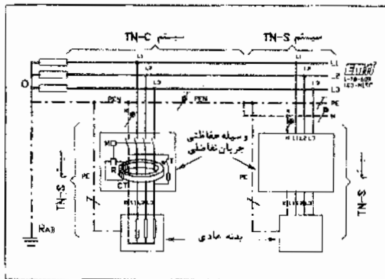
شکل ۲۲۱-۱۱ استفاده از وسایل حفاظتی جریان تفاضلی در سیستم TN-C-S
