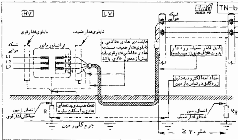
شکل 4P2 ۱۲. حالتی با دو اتصال زمین مجزا - کابل یا زره زمین شده و زمین تابلو از طریق PEN در سیستم TN
