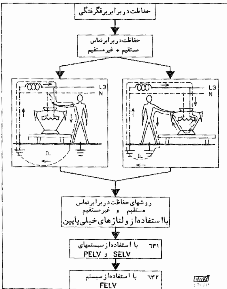
شکل ۱-۳۰- روشهای حفاظت در برابر هر دو نوع تماس - مستقیم و غیر مستقیم
