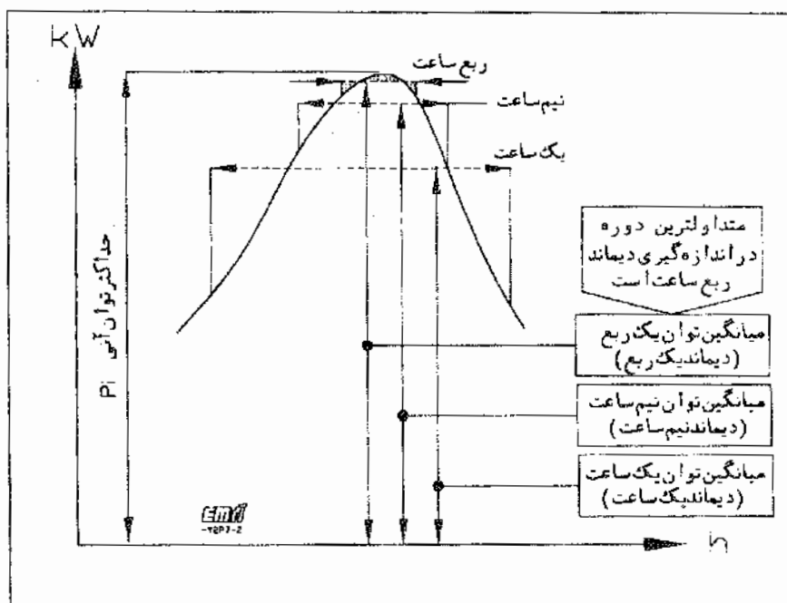
شکل 7P1-۲. قله منحنی بار در زیر ذره بین - هر چه دوره دیماند طولانی تر باشد، توان میانگین یا دیماند نسبت به حداکثر توان آبی کوچکتر می شود.
