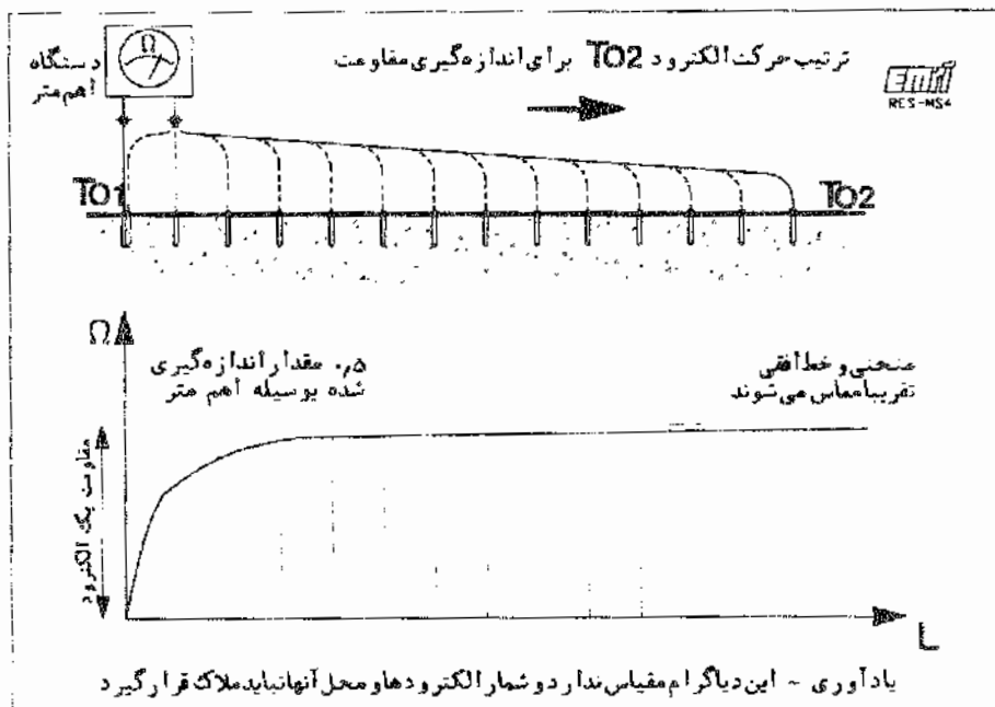
شکل ۴-۱- تغییرات مقاومت دو الکتروود نسبت به فاصله
