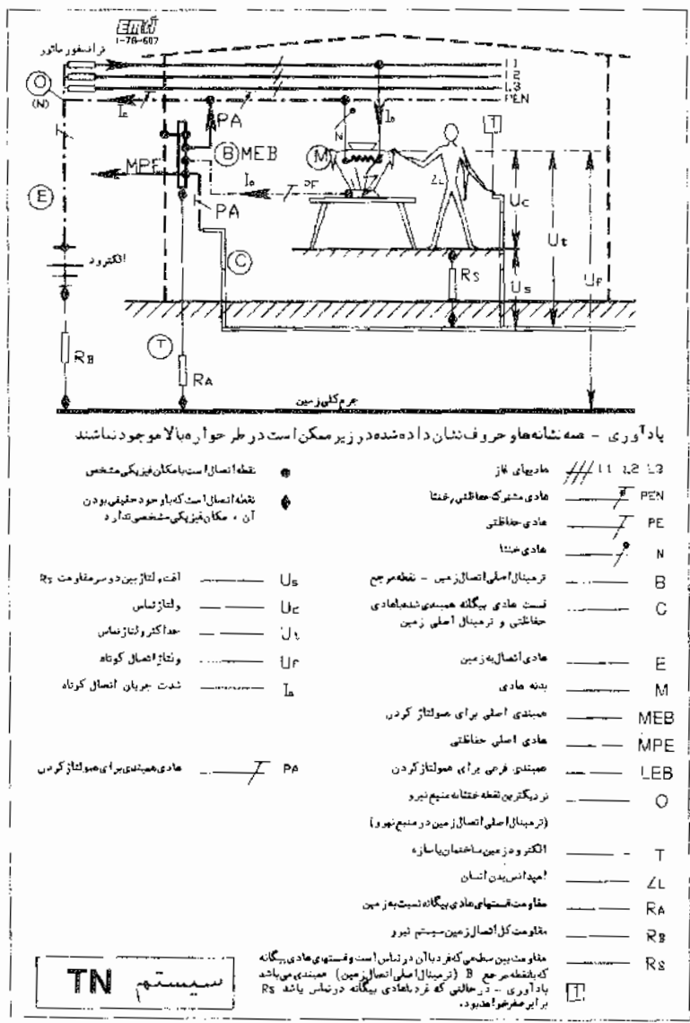
شکل ۶-۲۱ اجزای تشکیل دهنده یک سیستم معدنی اصلی برای همولتاژ کردن
