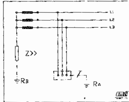
شکل ۳-۲۱۷ سیستم سه فاز نوع IT
