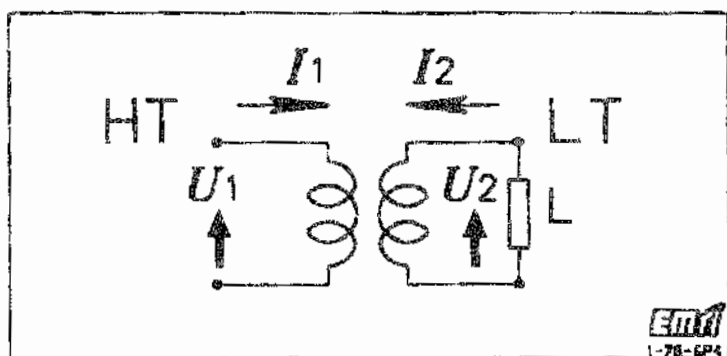
شکل ۸-6P4 حالتی که ترانسفورماتور بار اسمی را تغذیه می کند.
