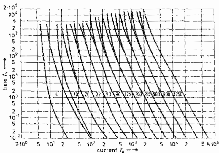
شکل ۴-6P4 منحنیهای جریان / زمان برای فیوزهای نوع gG طبق IEC 269
