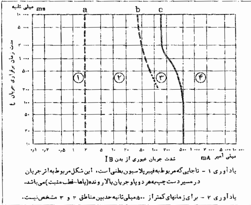
شکل ۱-۵۳۴ حوزه بندی نوع اثر جریان مستقیم
