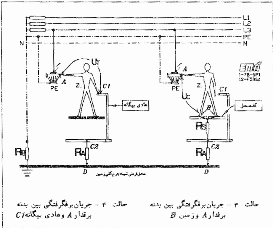
شکل ۲-6P1 برق گرفتگی در حالت‌های "تماس غیر مستقیم"
