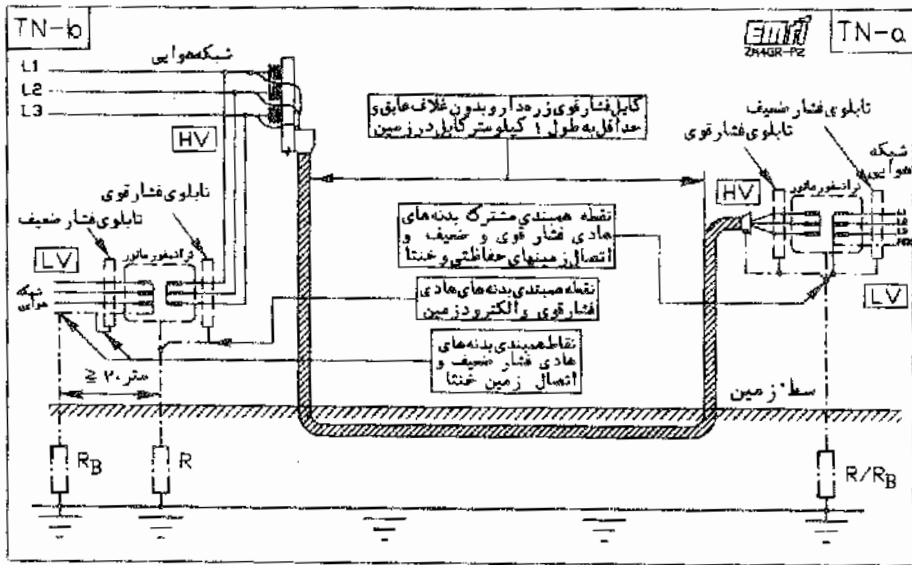
شکل 4P2-8 دو حالت مختلف برای احداث اتصال زمین - یکی مشترک و دیگری مجزا در سیستم TN
