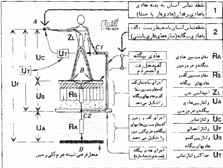
شکل 6P1-4 زنجیره مدار برگرفتگی - مقاومتها و ولتاژها
