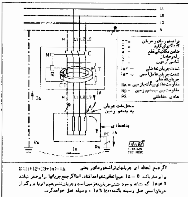
شکل ۲۲۱-۱۰ طرحواره یک وسیله (کلید) حفاظتی جریان تفاضلی
