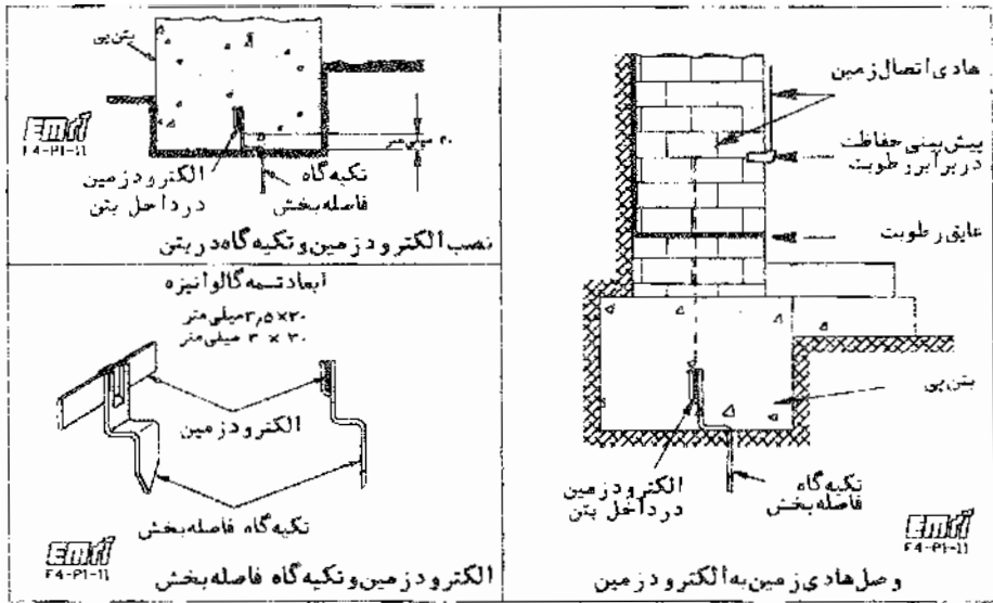
شکل ۲۱- 4PI- نحوه نصب الکترو د در داخل بتن
