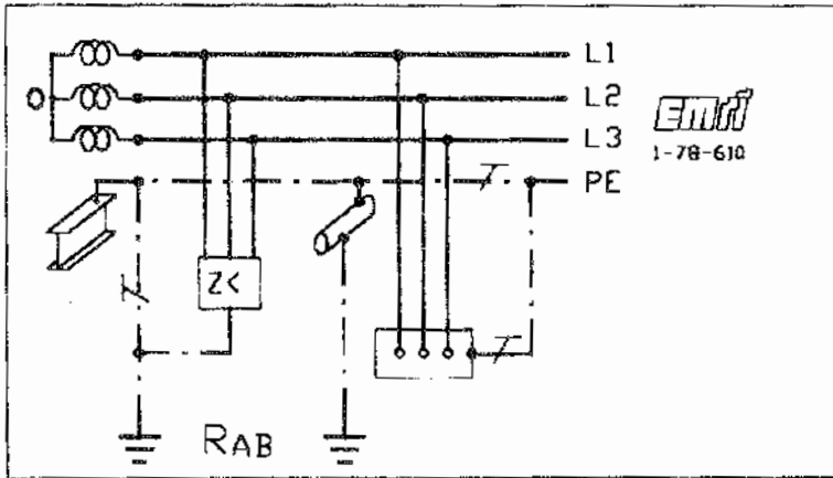
۶۲۱-۱۴-۴) سیستم IT مجهز به وسیله کشف اولین اتصال در خطای مصنوعی
