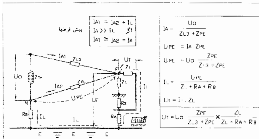
شکل ۲۰۳۴۱ جریانهها و ولتاژهای اتصال کوتاه و برقگرفتگی مربوط به حالت خاص شکل ۱-۲۴۱
