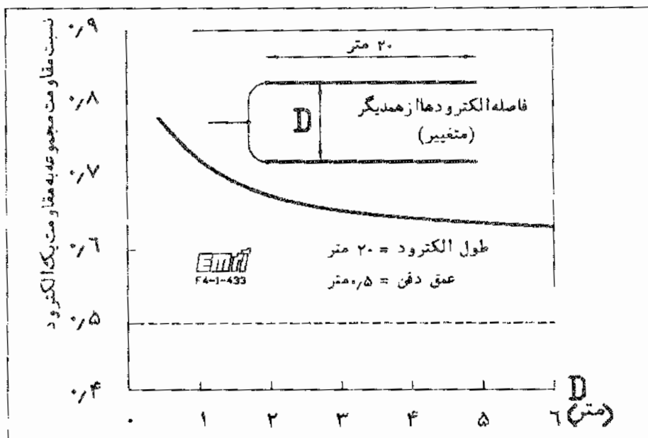
شکل ۴-۳۳-۲ تاثیر فاصله روی مقاومت کل دو الکترودهای افقی
