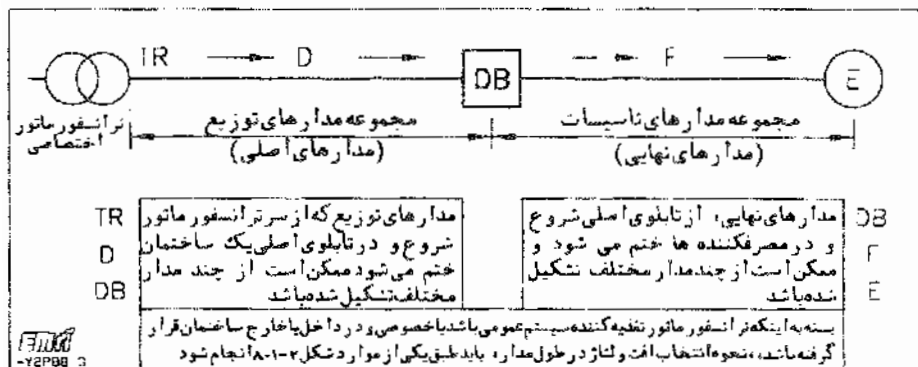
شکل ۸-۱-۱ طرحواره نحوه تقسیم افت ولتاژ بین مدارهای مختلف
