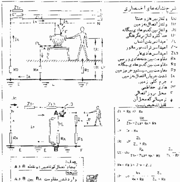
شکل ۲-۳۳۱ سیستمی که در آن علاوه بر نقطه ختای بدنه تجهیزات نیز به زمین وصل اند.
