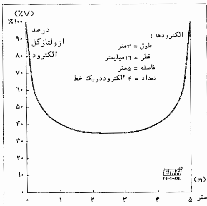
شکل ۳-۴۸۱ پتانسیل روی سطح زمین بین دو الکتروود و سطحی از چهار الکتروود در یک خط
