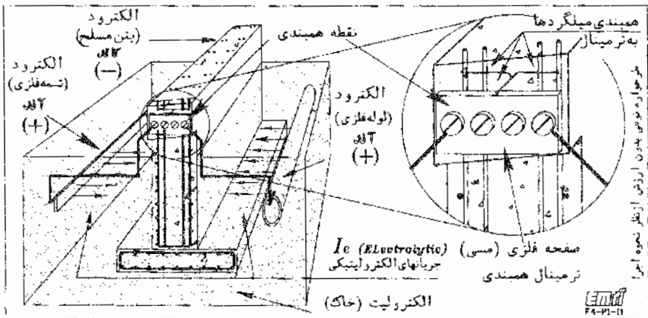
شکل 4P1-31-1 همبندی در تأسیسات اتصال زمین و تشکیل پیل گالوانیک
