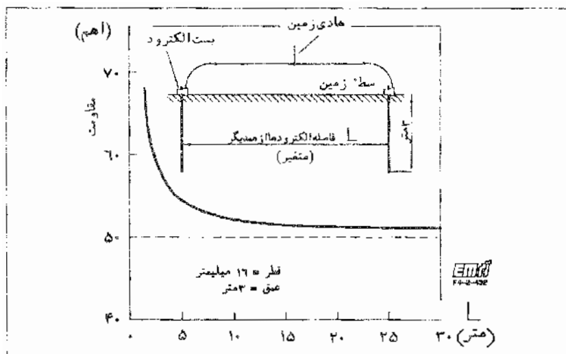
شکل ۴-۲-۲ مقاومت کل دو الکترود میله ای موازی با توجه به فاصله جدایی آنها
