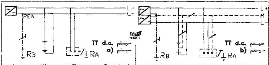
شکل ۲۱۸-۴ سیستم TT d.c.
