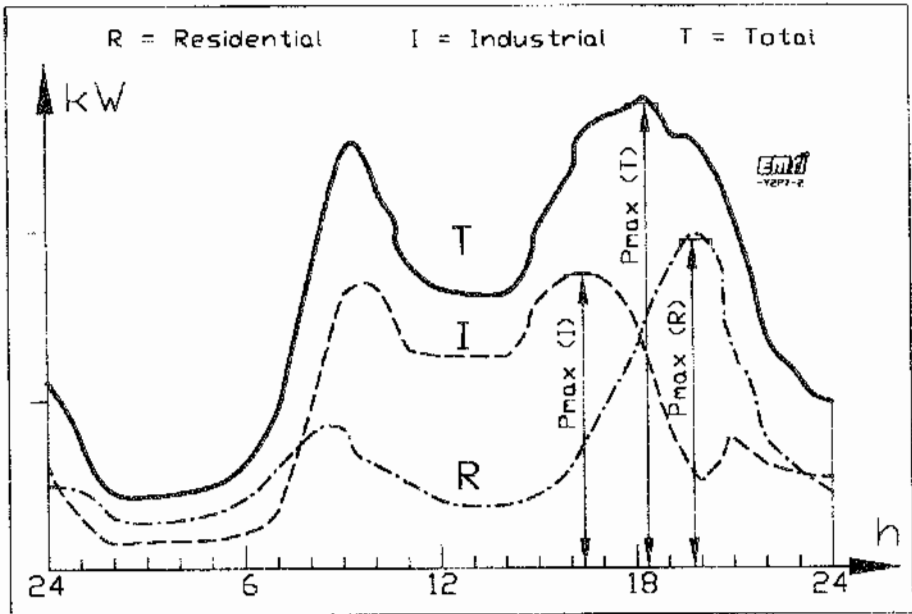
شکل 7P1-1 در هر لحظه توان کل T برابر است با مجموع توانهای حاصل از دو منحنی بار خانگی R و بار صنعتی I
