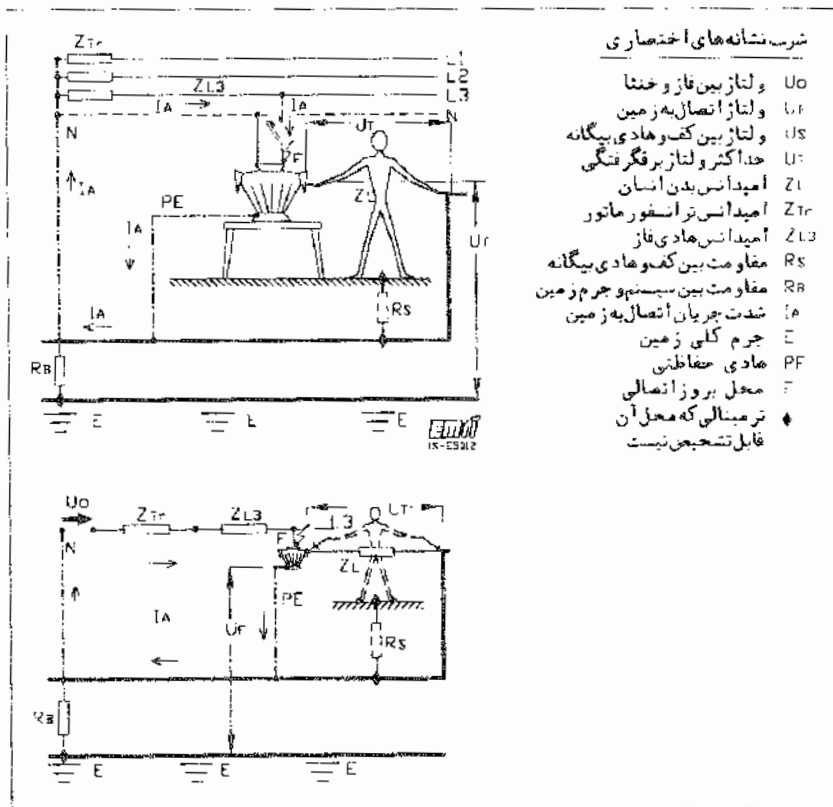
شکل ۳۳۳-۴ طرحواره یک سیستم اتصال "زمین" مصنوعی
