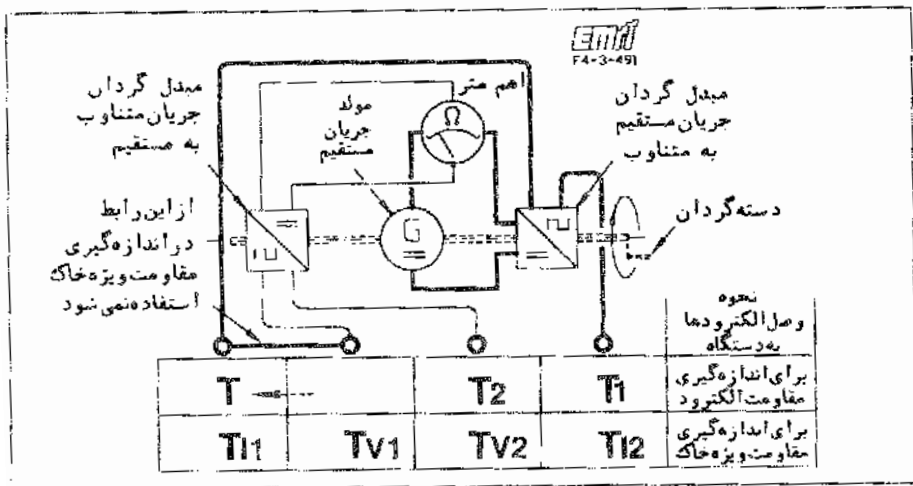
شکل ۳-۴۹۱ مدار یکی از وسایل اندازه گیری مقاومت الکتروود و مقاومت ویژه خاک
