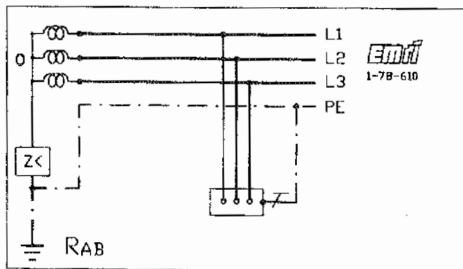
شکل ۱۴-۶۲۱ (۳) سیستم IT مجهز به وسیله کشف اولین اتصالی (نصب شده در ختای)
