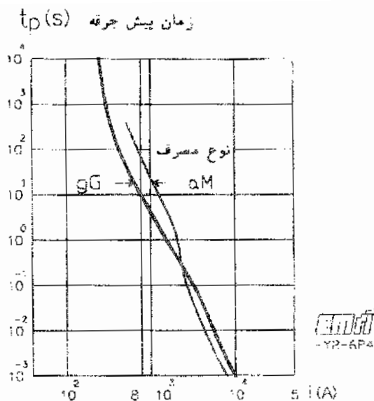
شکل ۶- 6P4-۴ منحنیهای دو فشنگ فیوز با جریان اسمی ۲۰۰ آمپر
