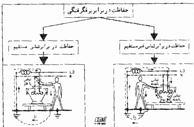
شکل ۶-۳-۱-۱ دو نوع برقگرفتگی و لزوم ایجاد شرایط ایمن در برابر آنها
