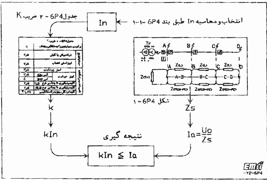
شکل 6P4-6 خلاصه نحوه کنترل کارایی سیستم با استفاده از ضریب K (روش انجام کار از روی ناچاری)
