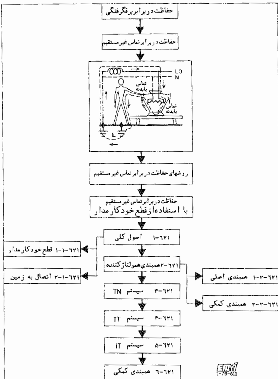
شکل 1-621 حفاظت در برابر تماس غیر مستقیم با قطع خودکار تغذیه، مهمترین موضوع در مبحث حفاظت است (بر اساس IEC 364-4-41)
