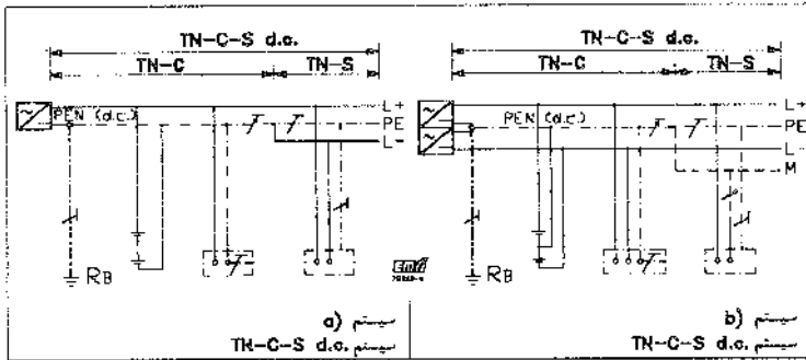
شکل ۲۱۸-۳ سیستم TN-C-S d.c.
