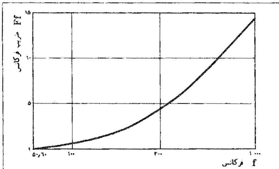
شکل ۳-۵:۱ تغییرات در آستانه فیبربلاسیون بطنی با پیچند فرکانس ۶۰/۵۰ تا ۱۰۰۰ هرتز و زمانی بیش از یک پرئود قلب و مسیر جریان در طول بدن
