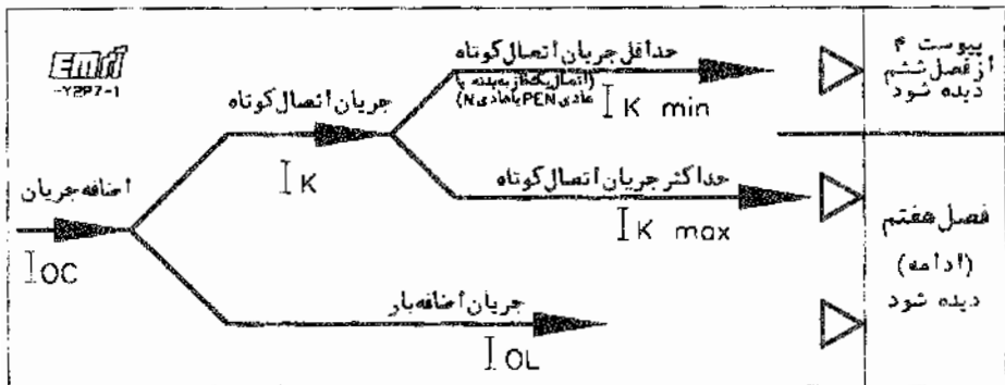
شکل ۲-۷۰۰ اضافه جریان و جریانهای اضافه بار و اتصال کوتاه به صورت طرحواره
