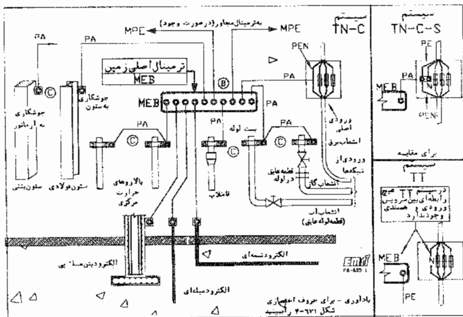
شکل ۶-۲۱ طرحواره یک نمونه همبندی برای همولتاژ کردن در سیستم (TT) TN
