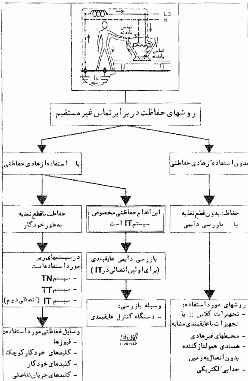
شکل ۱-۲۲۰ روشهای حفاظت در برابر تماس غیر مستقیم
