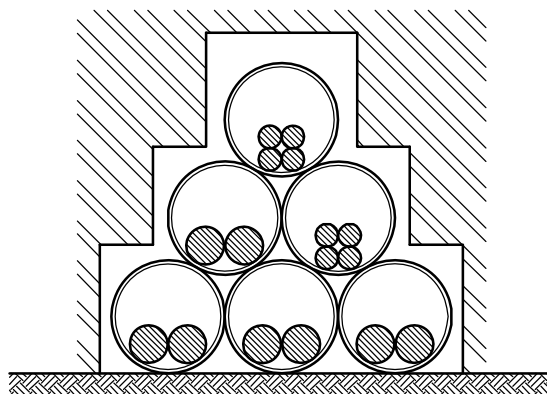
آرایش لوله و کابل فشار متوسط (Sc: 1:10)
