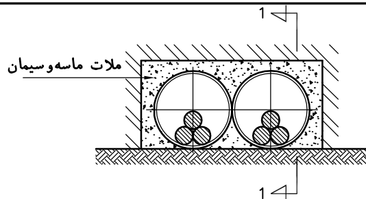
آرایش لوله و کابل فشار متوسط (Sc: 1:10)
