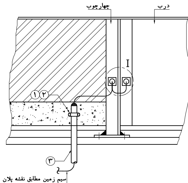
درب پست (Sc: N.T.S)
