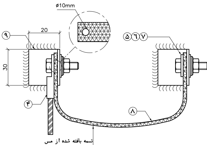
جزئیات I (Sc: N.T.S)
