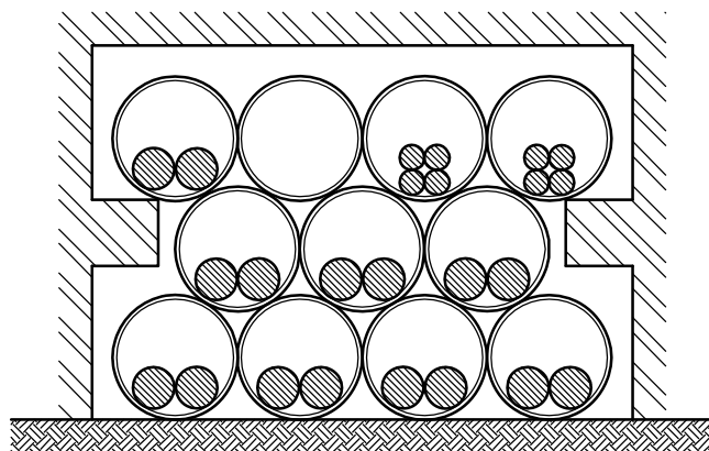
آرایش لوله و کابل فشار ضعیف در پست دوقاتی (Sc: 1:10)
