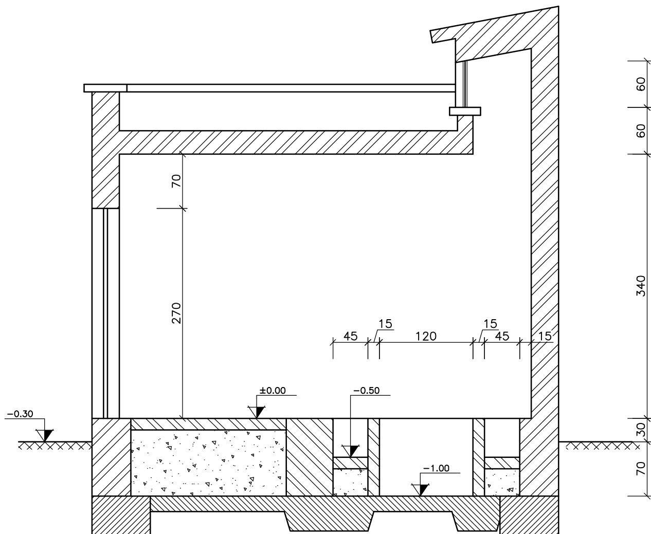
برشی B-B (Sc: 1:50)
