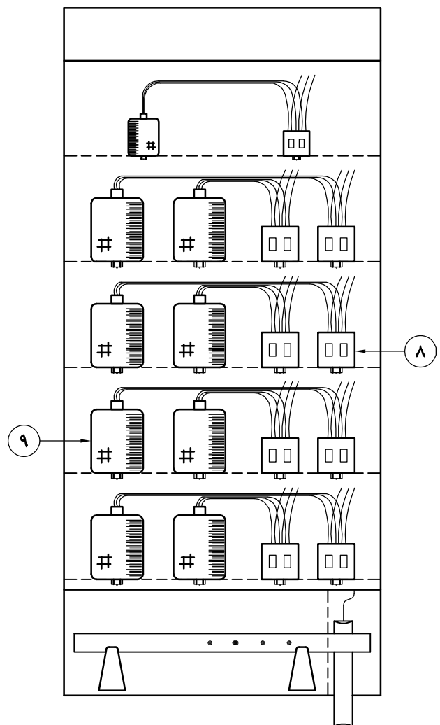
نمای داخلی تابلو از پشت
