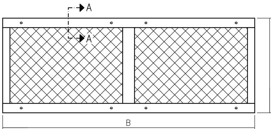
پلان بازو و فونداسیون کف
