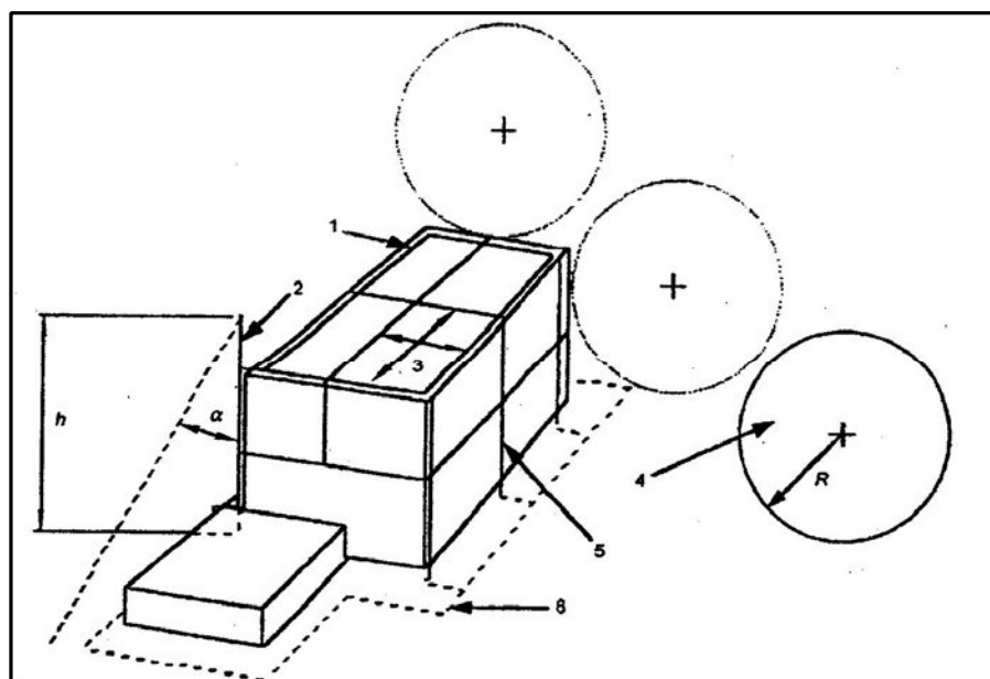
شکل (۱۱ b-۱۱): طرح سیستم حفاظتی با استفاده از اجزاء مختلف پایانه هوایی
